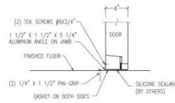
FLUSH DOOR JAMB ALUMINUM ANGLE
