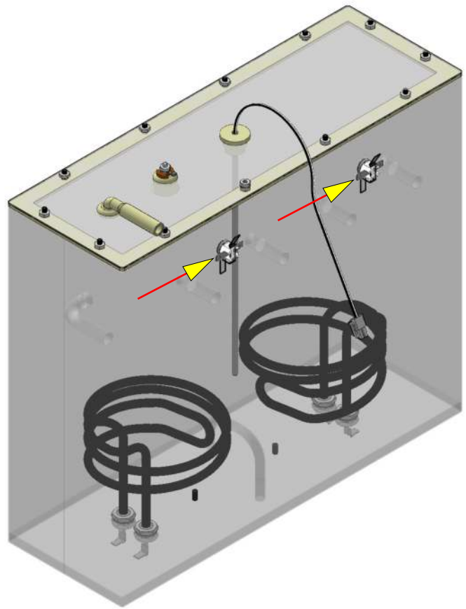
FIG. 18-2 LIMIT THERMOSTATS
