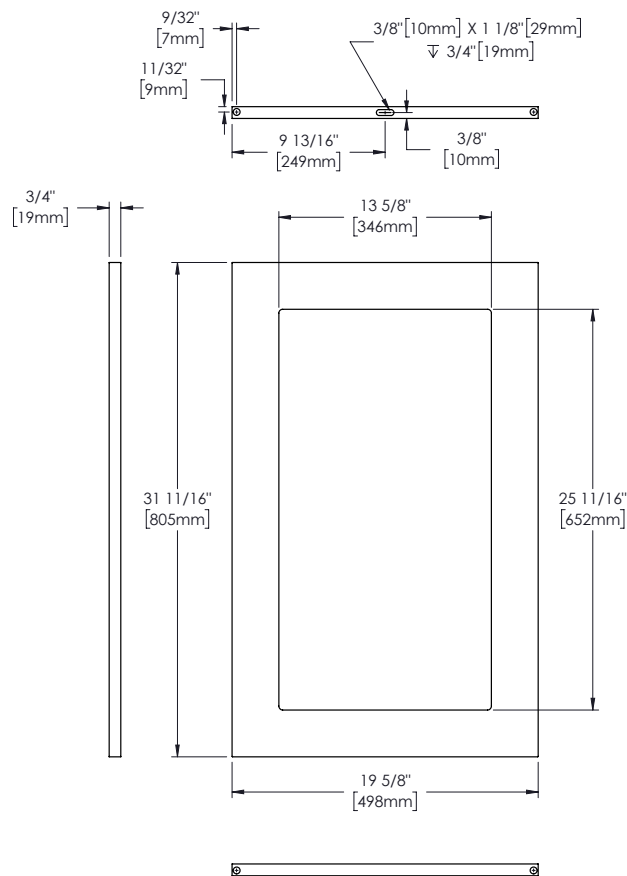
GLASS DOOR
